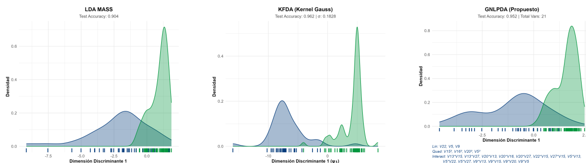
Figura 5.22: Comparativa geométrica de los espacios de proyección para el conjunto de datos Ionosphere.
