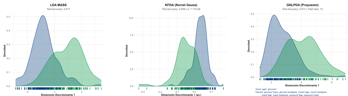
Figura 5.42: Comparativa geométrica de los espacios de proyección para el conjunto de datos Pima diabetes.
