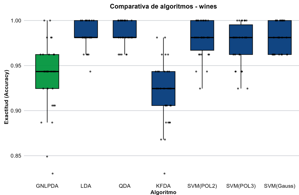
Figura 5.13: Distribución empírica del rendimiento predictivo para el conjunto de datos Wines.
