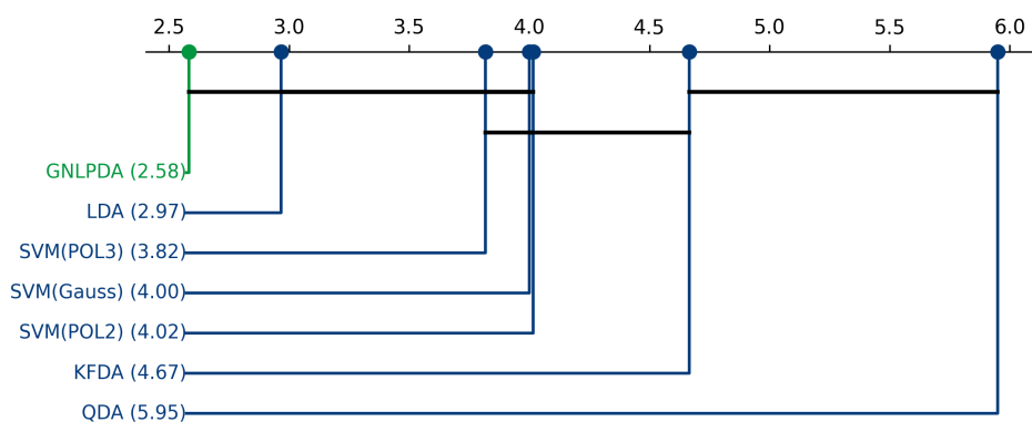
Figura 5.44: Análisis de significancia estadística post-hoc mediante distancias críticas de Nemenyi para el conjunto de datos pima diabetes.
