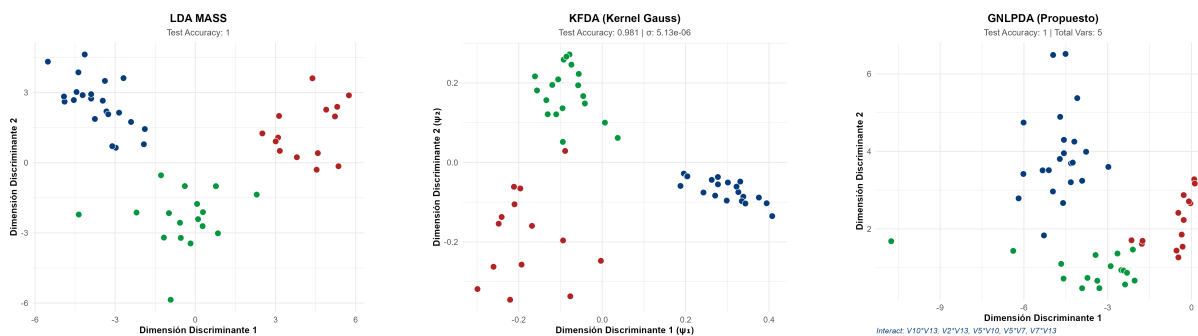
Figura 5.12: Comparativa geométrica de los espacios de proyección para el conjunto de datos Wines.
