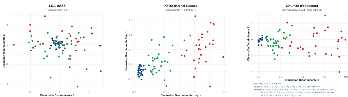
Figura 5.37: Comparativa geométrica de los espacios de proyección para el conjunto de datos cebolla 20D.
