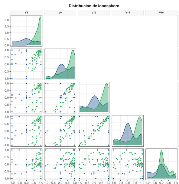
Figura 5.21: Gráficos de dispersión por pares de Ionosphere .
