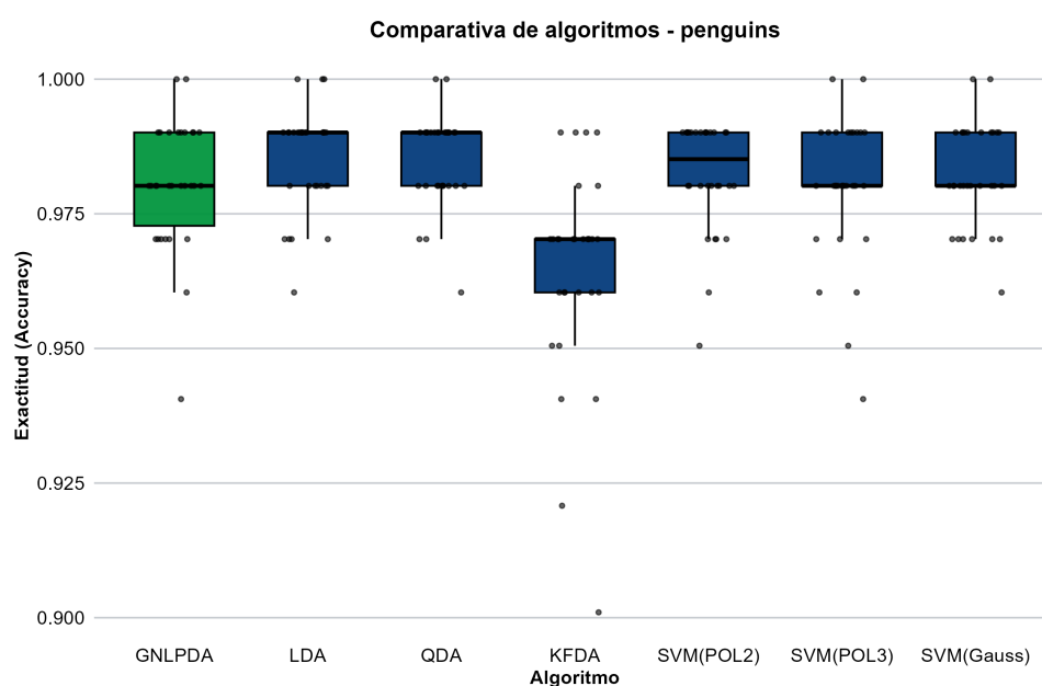
Figura 5.8: Distribución empírica del rendimiento predictivo para el conjunto de datos Penguins.
