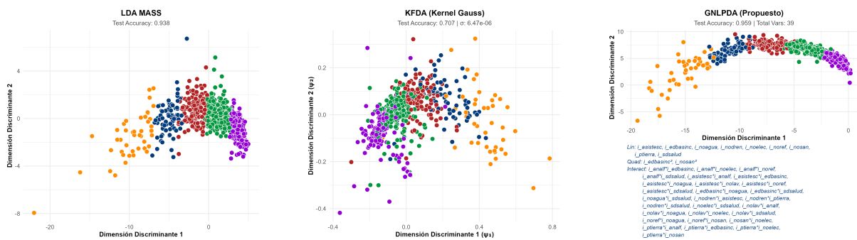
Figura 5.53: Comparativa geométrica de los espacios de proyección para el conjunto de datos Indicadores 2020 (2D).
