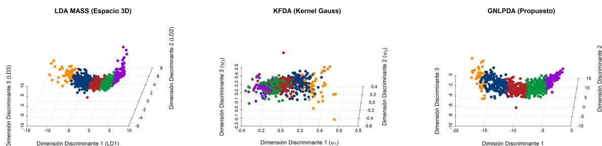
Figura 5.48: Comparativa geométrica de los espacios de proyección para el conjunto de datos Indicadores 2015 (3D).
