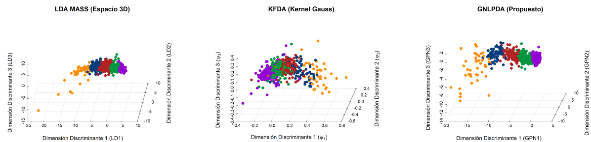
Figura 5.54: Comparativa geométrica de los espacios de proyección para el conjunto de datos Indicadores 2020 (3D).
