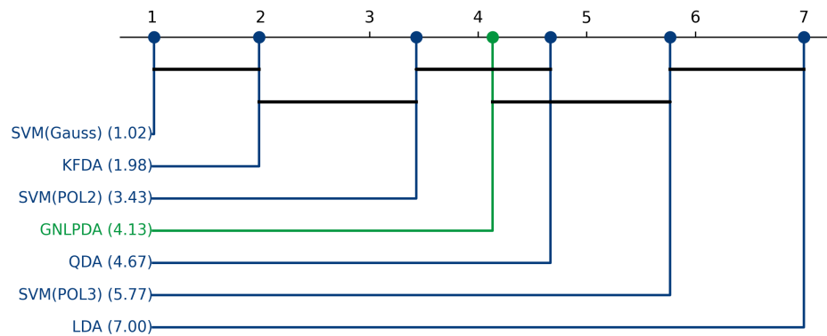
Figura 5.39: Análisis de significancia estadística post-hoc mediante distancias críticas de Nemenyi para el conjunto de datos cebolla 20D.
