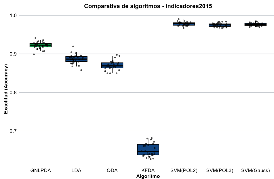
Figura 5.49: Distribución empírica del rendimiento predictivo para el conjunto de datos Indicadores 2015.
