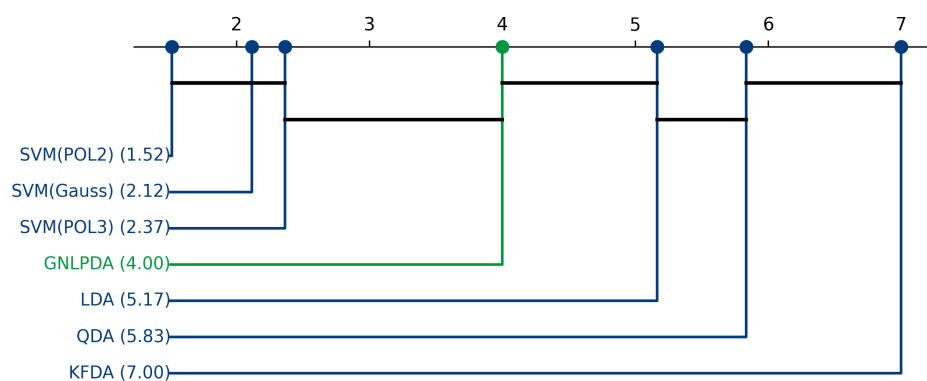
Figura 5.50: Análisis de significancia estadística post-hoc mediante distancias críticas de Nemenyi para el conjunto de datos Indicadores 2015.
