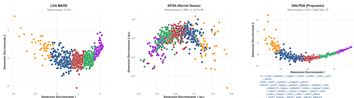
Figura 5.47: Comparativa geométrica de los espacios de proyección para el conjunto de datos Indicadores 2015 (2D).
