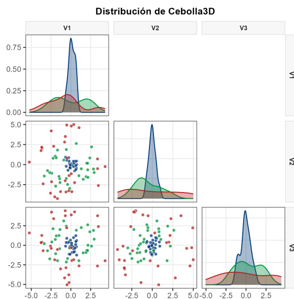
Figura 5.26: Gráficos de dispersión por pares de Cebolla3D.
