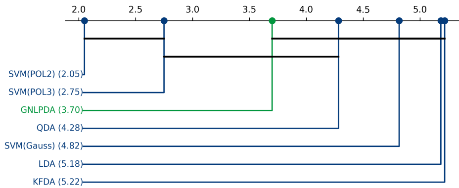
Figura 5.19: Análisis de significancia estadística post-hoc mediante distancias críticas de Nemenyi para el conjunto de datos Cancer Wisconsin.
