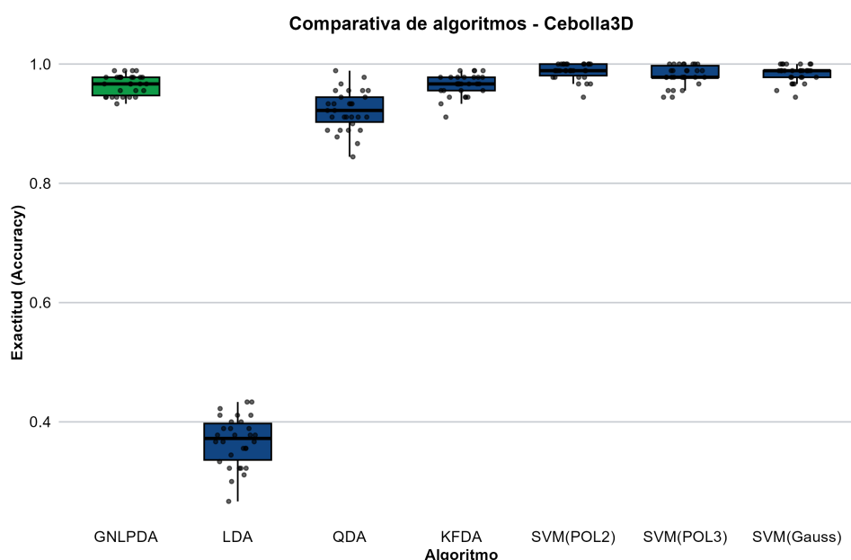
Figura 5.28: Distribución empírica del rendimiento predictivo para el conjunto de datos cebolla 3D.
