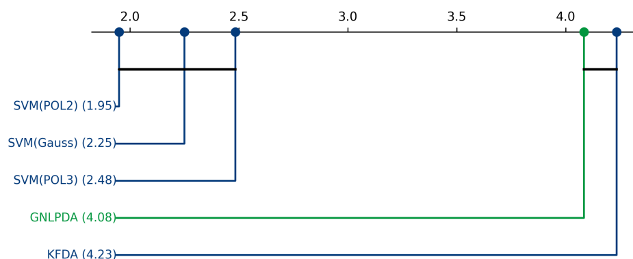
Figura 5.30: Análisis de significancia estadística post-hoc y corrección por enmascaramiento mediante distancias críticas de Nemenyi para el conjunto de datos Cebolla 3D.
