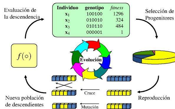
Figura 2.4: Diagrama de flujo del ciclo evolutivo de un algoritmo genético. Tomada de [76].
