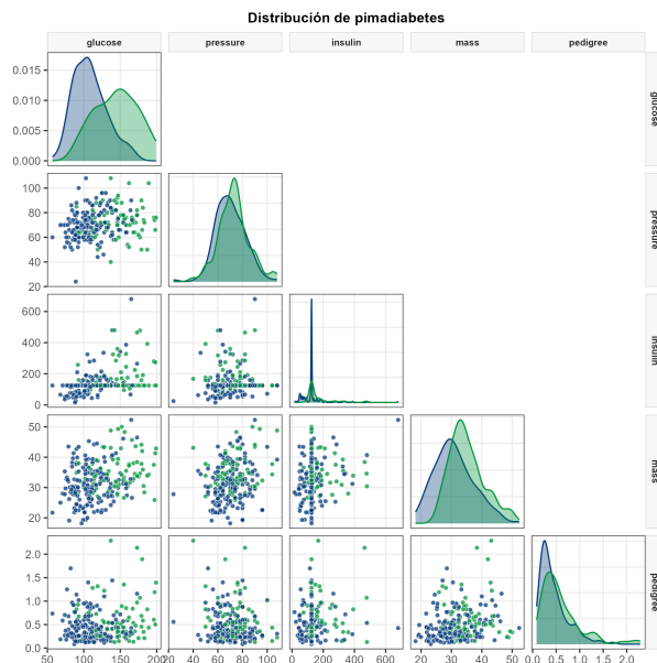
Figura 5.41: Gráficos de dispersión por pares de Pima Diabetes
