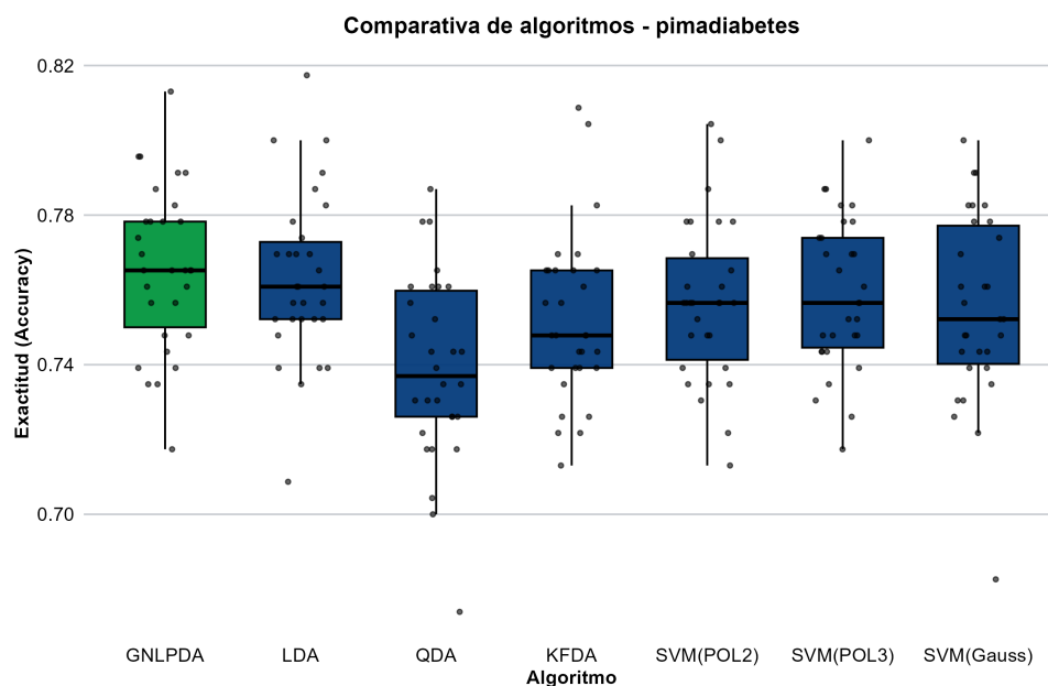
Figura 5.43: Distribución empírica del rendimiento predictivo para el conjunto de datos Pima diabetes.
