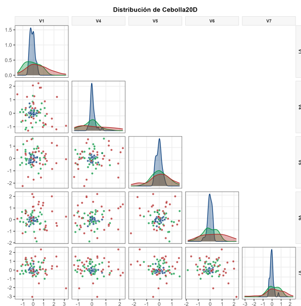
Figura 5.36: Gráficos de dispersión por pares de Cebolla20D.
