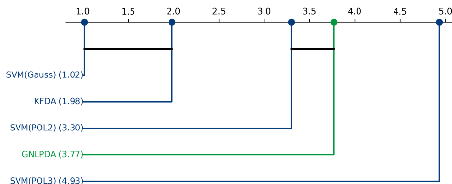
Figura 5.40: Análisis de significancia estadística post-hoc y corrección por enmascaramiento mediante distancias críticas de Nemenyi para el conjunto de datos cebolla 20D.
