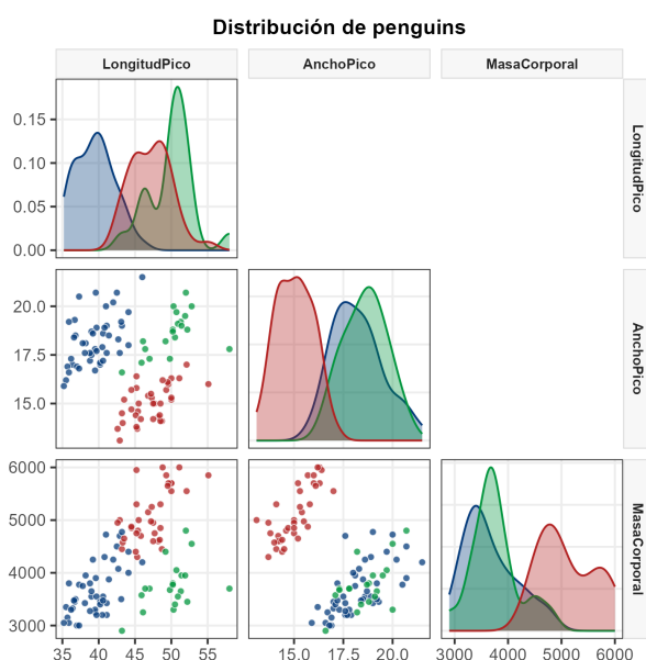
Figura 5.6: Gráficos de dispersión por pares de Palmer Penguins.
