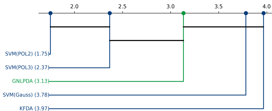
Figura 5.20: Análisis de significancia estadística post-hoc y corrección por enmascaramiento mediante distancias críticas de Nemenyi para el conjunto de datos Cancer Wisconsin.
