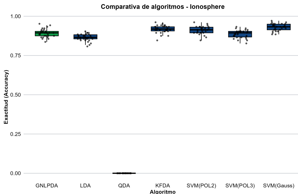
Figura 5.23: Distribución empírica del rendimiento predictivo para el conjunto de datos Ionosphere.
