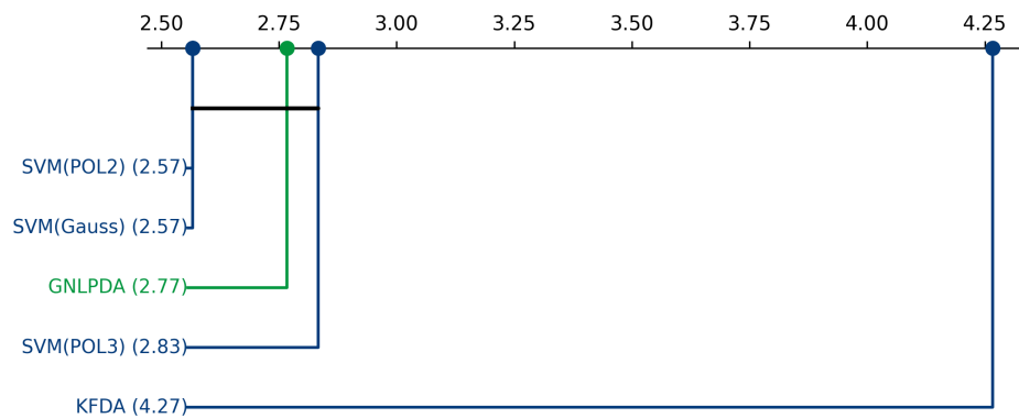
Figura 5.10: Análisis de significancia estadística post-hoc y corrección por enmascaramiento mediante distancias críticas de Nemenyi para el conjunto de datos Palmer penguins.
