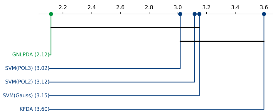
Figura 5.45: Análisis de significancia estadística post-hoc y corrección por enmascaramiento mediante distancias críticas de Nemenyi para el conjunto de datos Pima diabetes.
