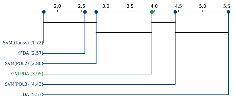
Figura 5.24: Análisis de significancia estadística post-hoc mediante distancias críticas de Nemenyi para el conjunto de datos Ionosphere.
